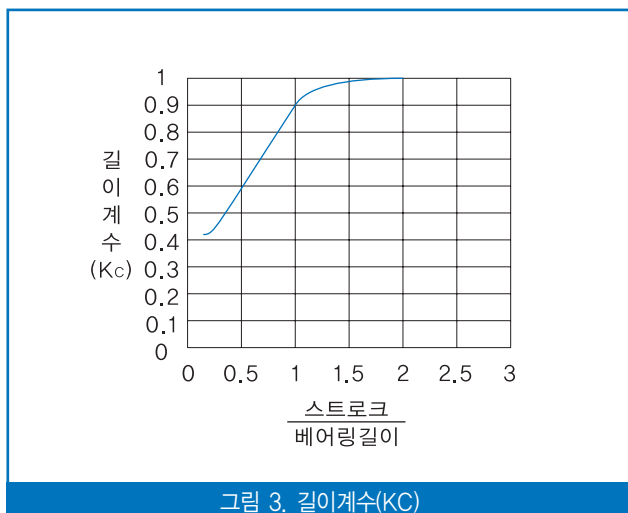
그림 3. 길이계수(KC)
