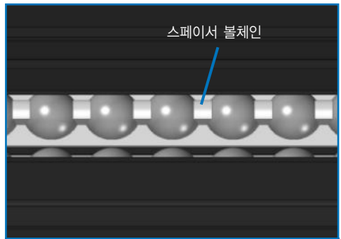
H-S시리즈 궤도부 상세
