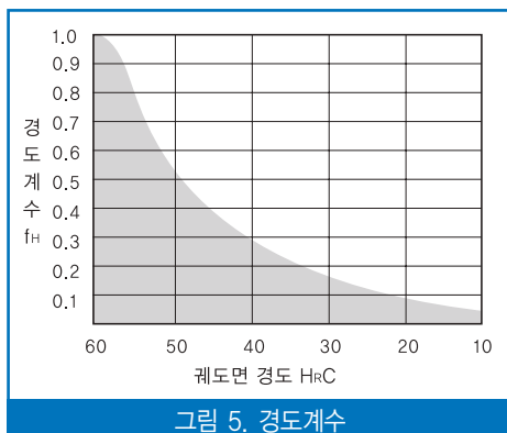
그림 5. 경도계수
