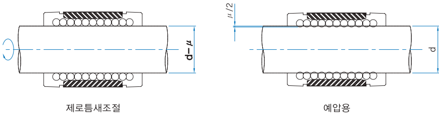
그림 4. 제로 틈새와 예압
