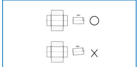
그림 15. LM샤프트를 삽입하는 방법 예
