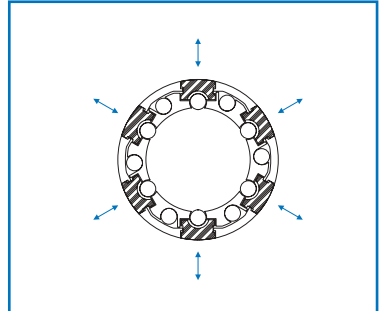
그림 3. 틈새조절
