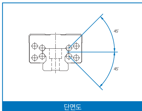
HS시리즈 (총볼타입)
