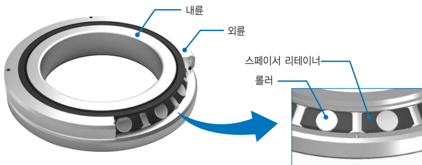
그림 1. 크로스롤러베어링 구조
