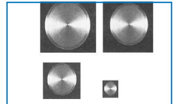
그림 2. 경화층사진
