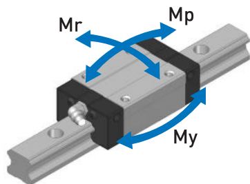
모멘트 강성
