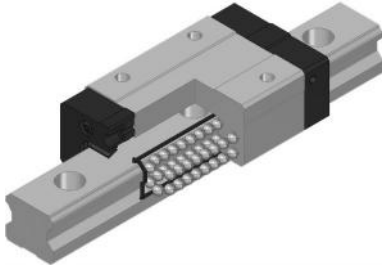
S시리즈 (총볼타입)
