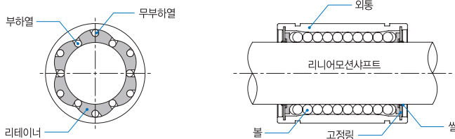
그림 1. WON 리니어볼부싱의 구조
