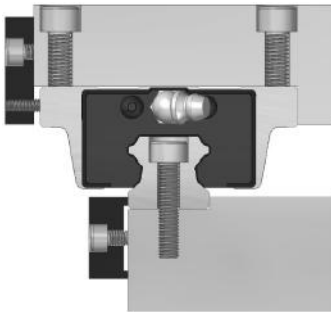
그림8. 측면 압력판 밀기 방식
