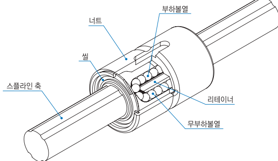
그림 12. 리니어 볼스플라인의 구조
