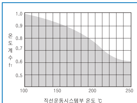
그림 6. 온도계수
