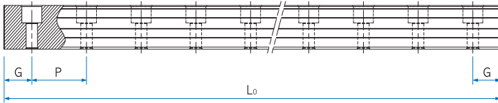
레일의 표준길이와 최대길이
