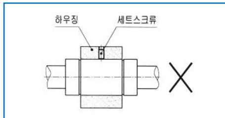
그림 8. 세트스크류 설치 예
