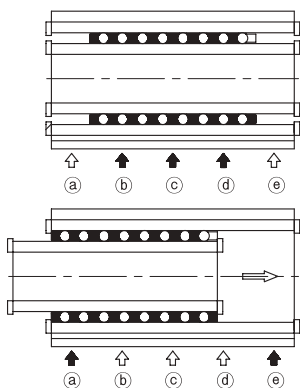
그림 5. 조정볼트의 체결 수순
