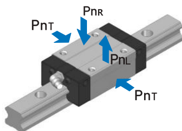
레이디얼 강성
