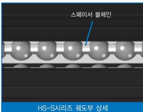
HS-S시리즈 (스페이서 체인타입)
