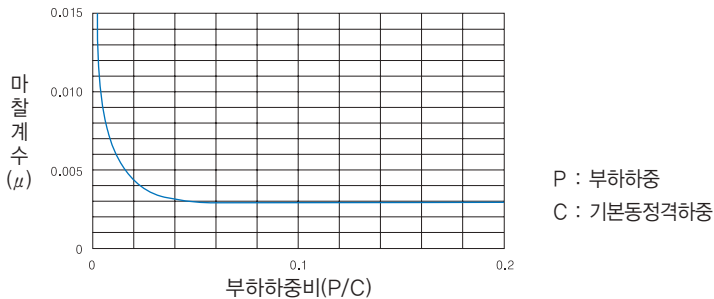
그림5. 부하하중비와 마찰계수의 관계
