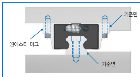
그림20. 기준축 리니어모션가이드
