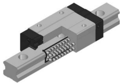
S-S시리즈 (스페이서 체인타입)
