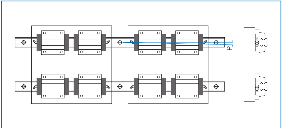
그림18. 2축 평행도 오차 허용치( P_1 )
