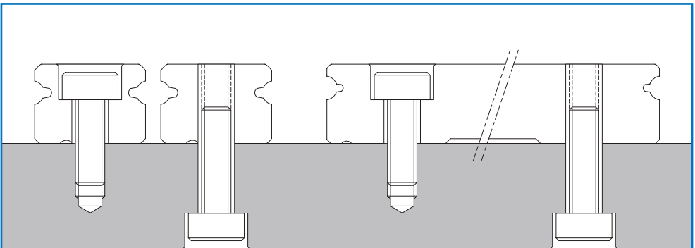
볼트체결
