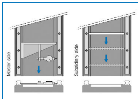
지그를 이용한 조립
