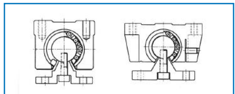
그림 11. 개방형 설치 예
