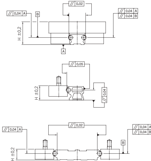
그림 2. 정도
