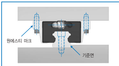
그림21. 중동축 리니어모션가이드
