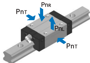
레이디얼 강성
