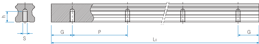
레일의 탭홀 타입 규격
