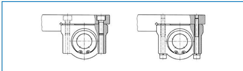
그림 13. 케이스 유닛의 설치
