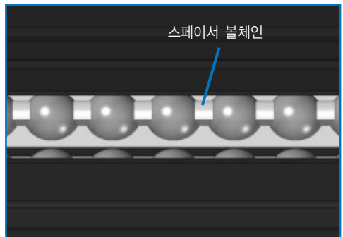
S-S시리즈 궤도부 상세
