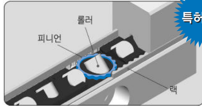
Anti-Creep 부상세도
