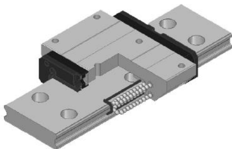
HW시리즈 (총볼타입)
