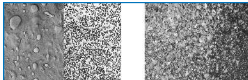
구상화 조직
