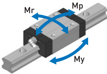
모멘트 강성
