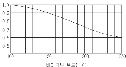
그림 2. 온도계수
