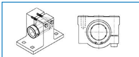
그림 10. 틈새조정형 설치 예
