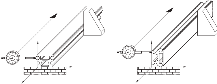
그림 1. 측정방법
