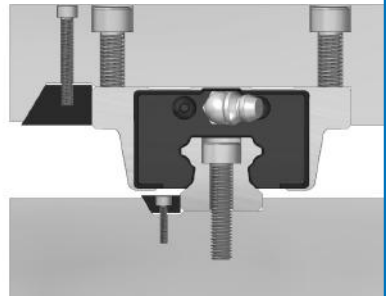
그림9. 테이퍼핀 밀기 방식
