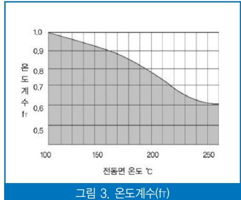
그림 3. 온도계수( f_T )
