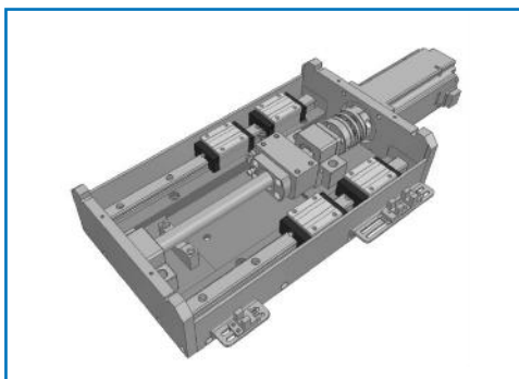
리니어모션가이드 설치 완성
